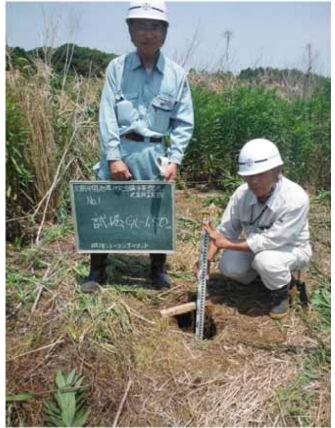
試験穴 GL-1.50 m
