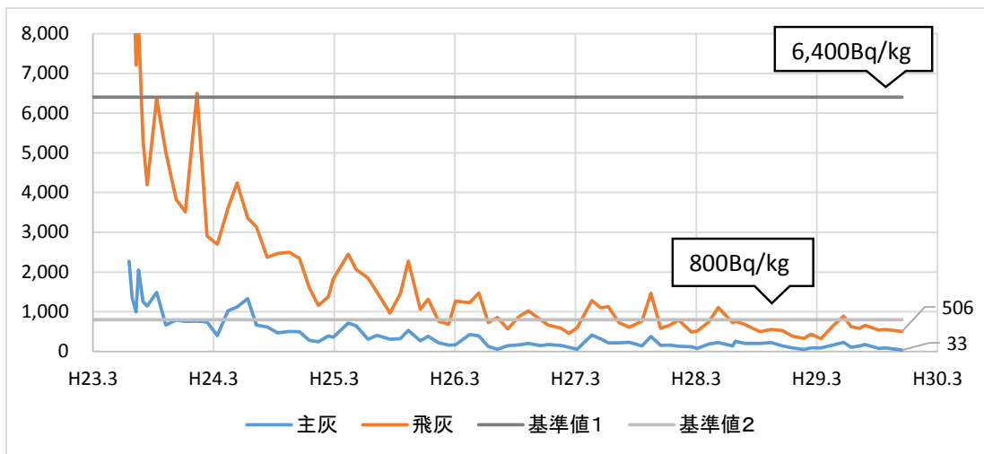
印西クリーンセンターにおける焼却灰放射能濃度測定値
